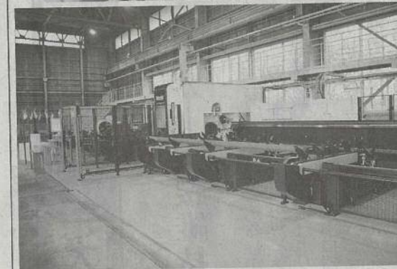
導入したヤマザキマザック製の3次元レーザー加工機「3Dファブリギア400Ⅲ」
